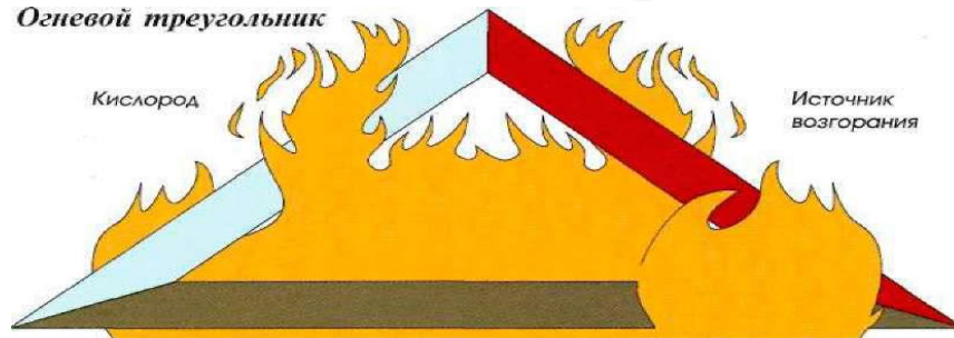
Огневой треугольник
